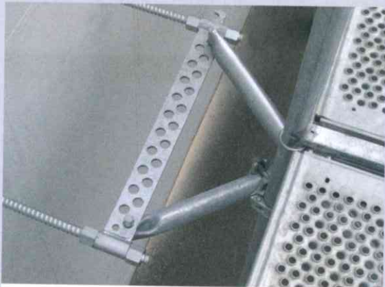
Kombination mit V-Anker
