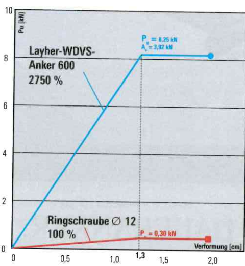
Vergleich Ringschraube mit WDVS-Anker
